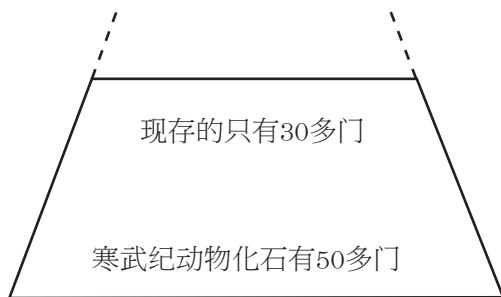
图25 寒武纪动物化石与现代物种之证据 寒武纪动物化石，门一级的有50多门，而现存的只有30多门。
