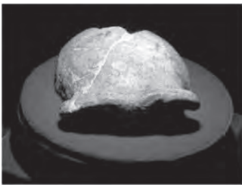
图47 所谓的“北京人”头盖骨公展 三维动画展示化石 （2003年9月22日，中国深圳新闻网）
