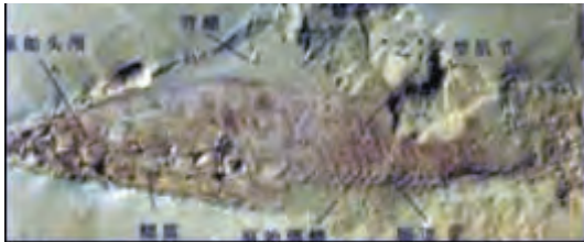
图12 世上已知最古老的脊椎动物“海口鱼”（ Haikouichthys ）化石（也被称为“世界第一鱼”） ( http://www.nsf.gov.cn/e_nsf/c/desktop/zl/cg/ddqq_016.htm )
