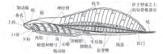
图15 世上已知最古老的脊椎动物“海口虫”模拟图 ( http://tech.tom.com/Archive/1121/1122/2002/8/5-32553.html )
