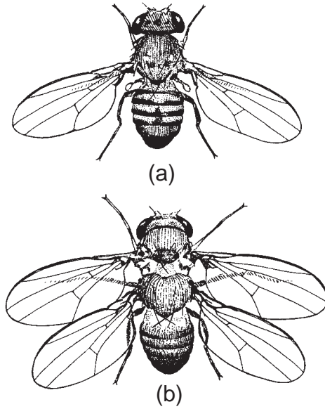
图61 正常果蝇和四翼果蝇
